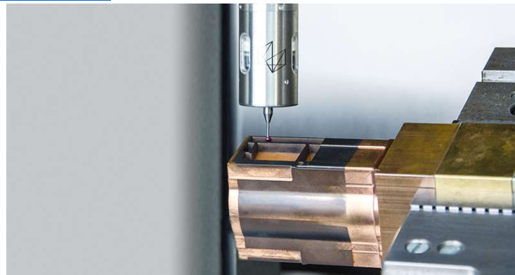
赤外線プローブ「IRP40.50」
