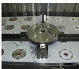
2 形状の異なるワークを同時にクランプして段取り削減
