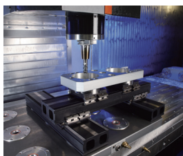
10 バイスにバイスを直行させた使用方法
