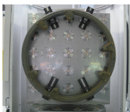
5 円形ワークをイケールに固定
