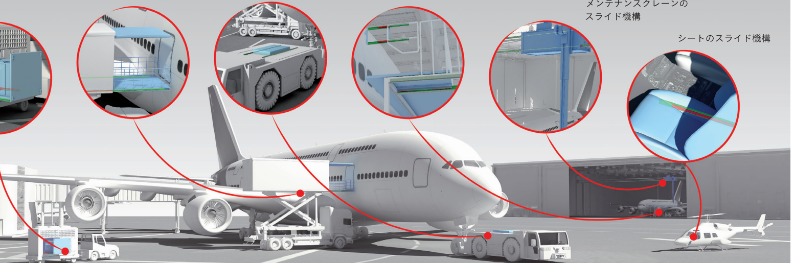
プラットホームの スライド機構
