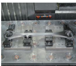
6 異型ワークも簡単に固定可能
