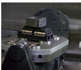
9 生材のクランプ“しろ”を極限まで抑えた強力爪
