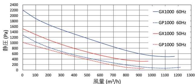
GX1000 GP1000 性能曲線
